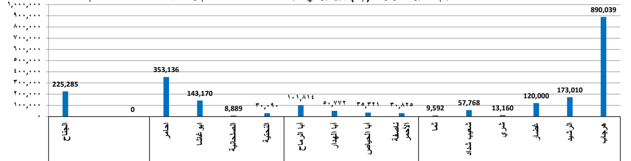
حجم السيول الواردة (م ٣ ) بين يومي الجمعة ٢٩/٤/٢٠٢٢م و السبت ٣٠/٤/٢٠٢٢م
